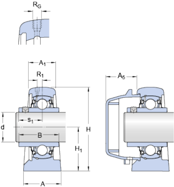
Bearing No. SYFWR 20 YTHR
