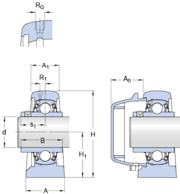
Bearing No. SYFWR 1.3/16 YZTHR
