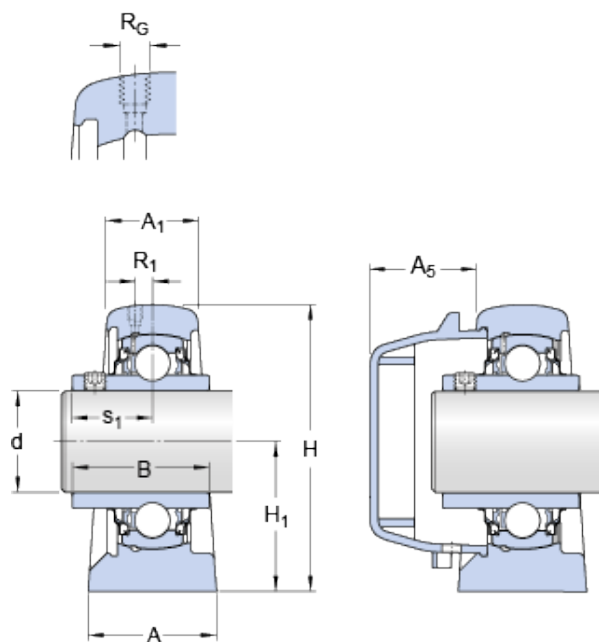
Bearing No. SYFWR 1.1/2 YZTHR
