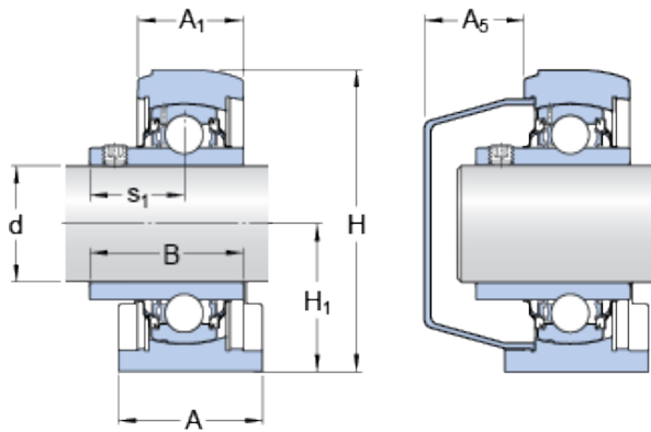
Bearing No. SYFWK 40 LTA
