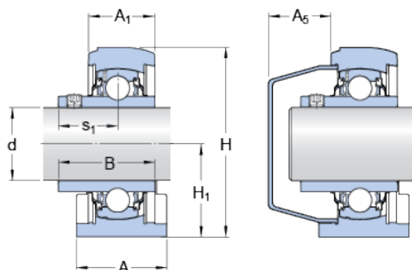
Bearing No. SYFWK 1.3/16 LTHR
