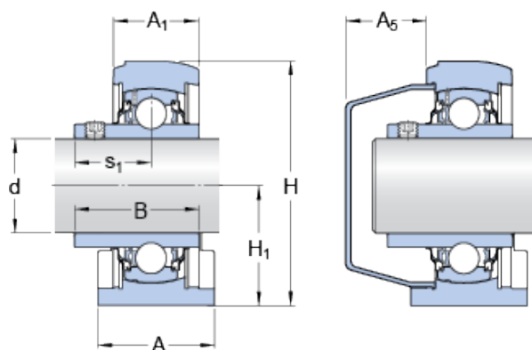
Bearing No. SYFWK 1.1/4 LTA
