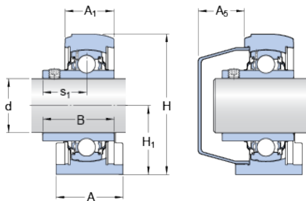
Bearing No. SYFWK 1.1/4 ALTHR
