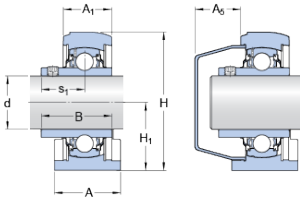
Bearing No. SYFWK 1.1/2 LTHR
